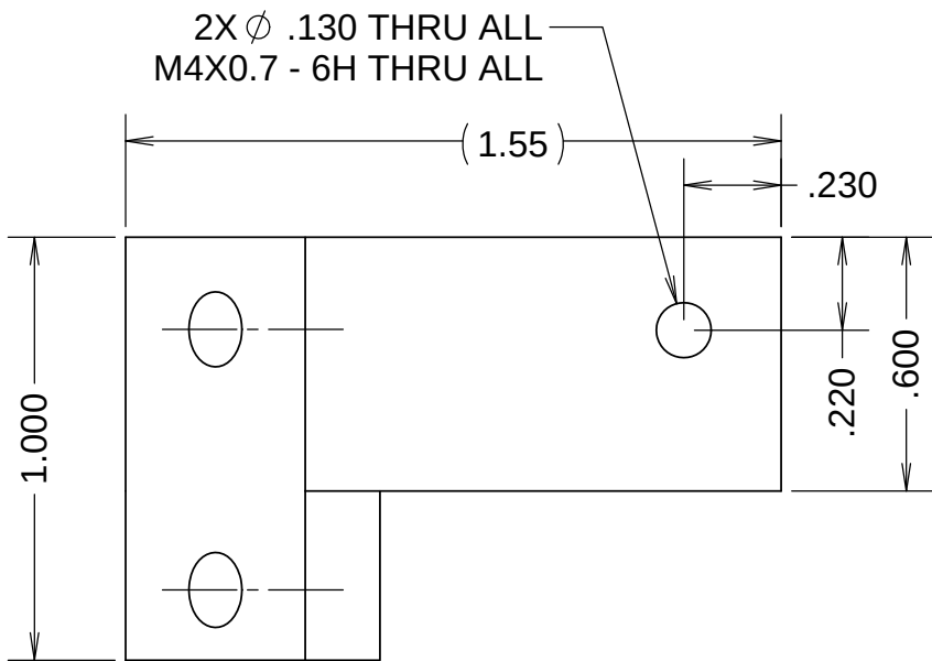
VIEW A-A
